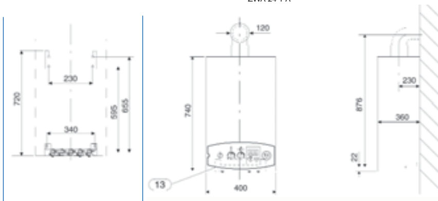
Piastra di allacciamento e staffa di sostegno
